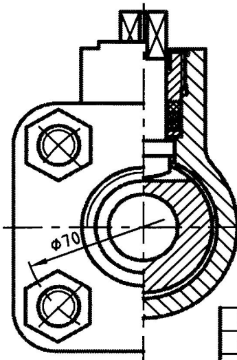
A-A 拆去扳手13
